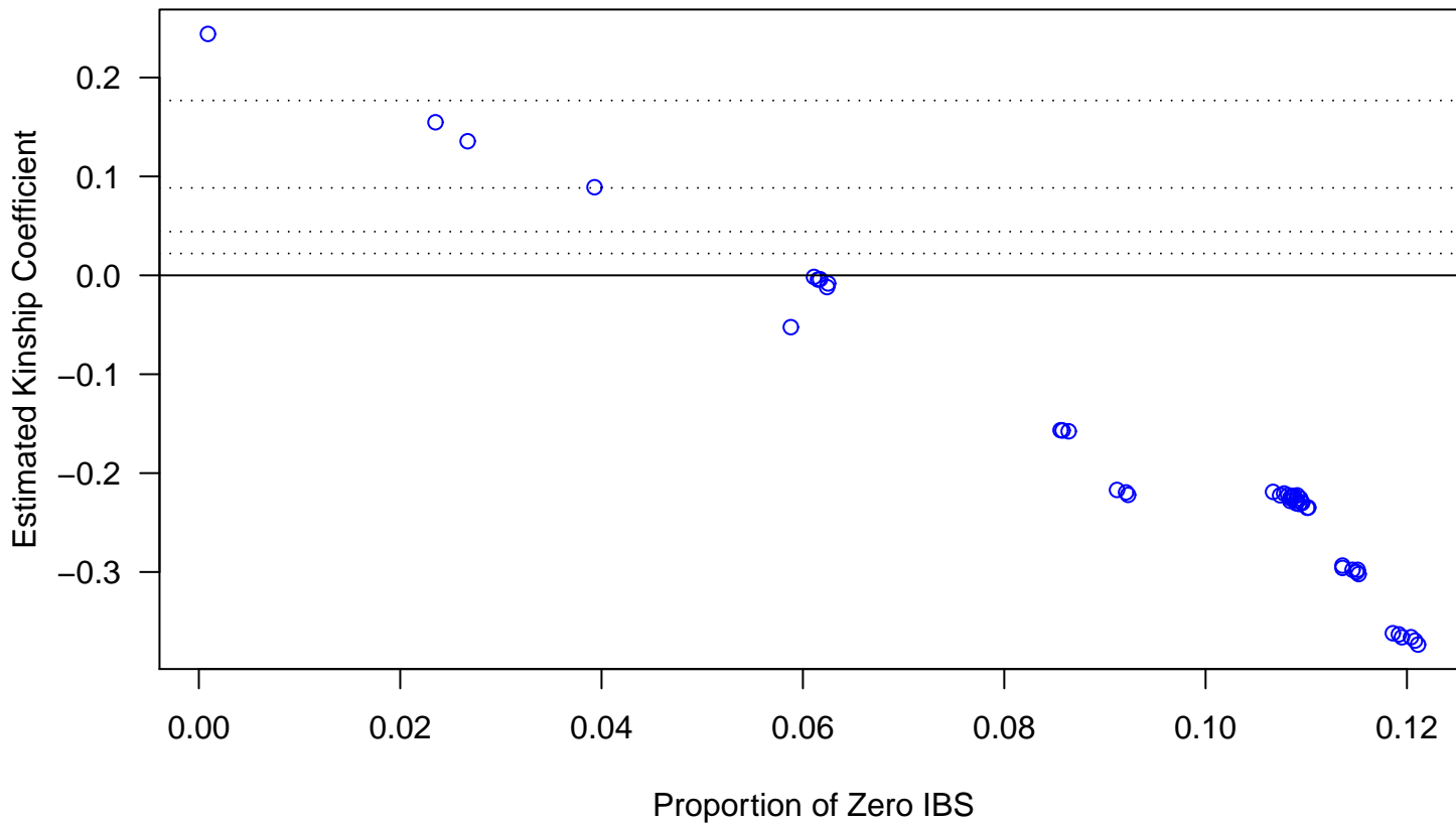
KING-Robust (Default)
